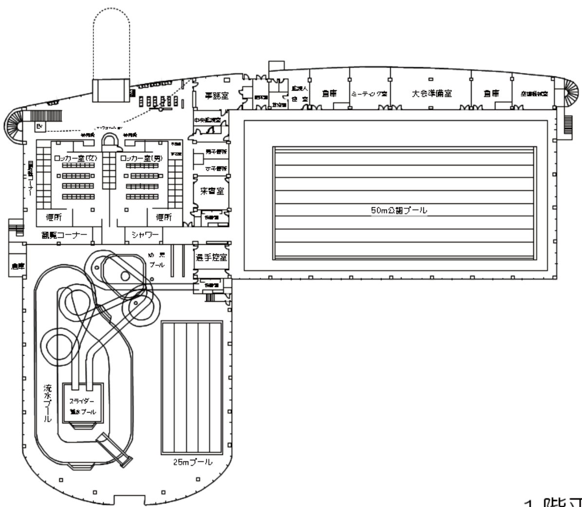
1階平面図
